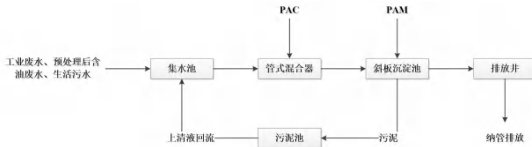
图 9.2-1 综合废水处理站工艺流程图
