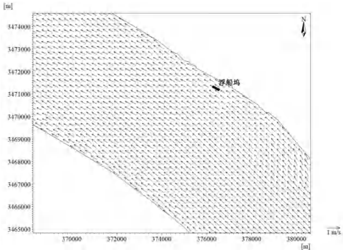
图 6.2.3-9 工程后涨急流场图
