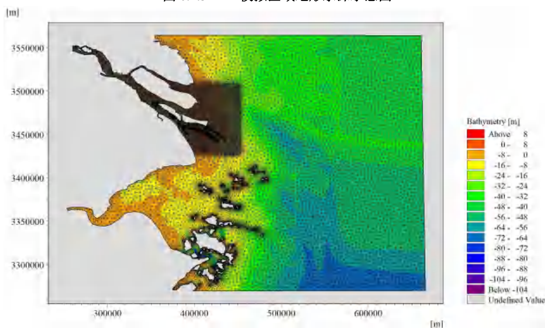
图 6.2.3-2 模拟区域网格划分示意图
