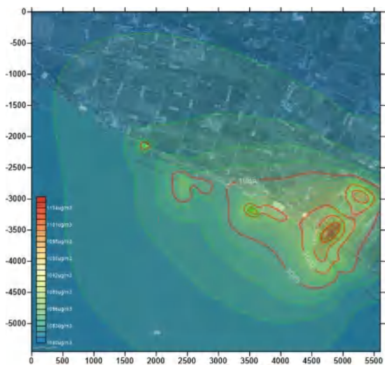
图 6.1-7 叠加现状后 VOCs 小时平均浓度分布图
