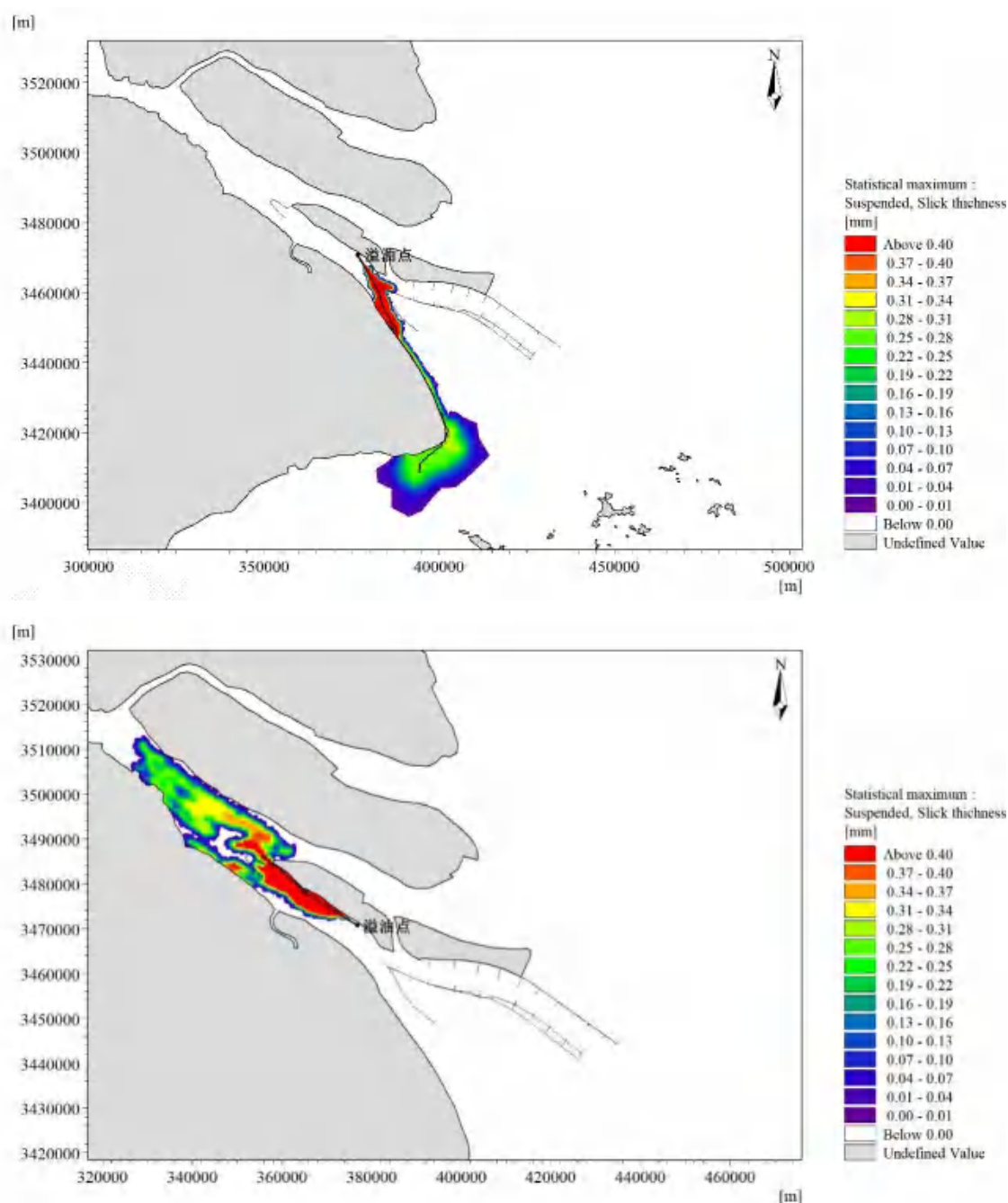
图 8.7.1-4 不利风向作用下油膜扫海面积和漂移轨迹图 (上为丰水期 WNN 风向落潮溢油，下为枯水期涨潮 ESE 风向溢油，48h)
