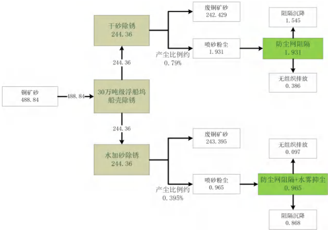
图 4.2.3-6 本工程砂料物料平衡图 (单位: t/a)
