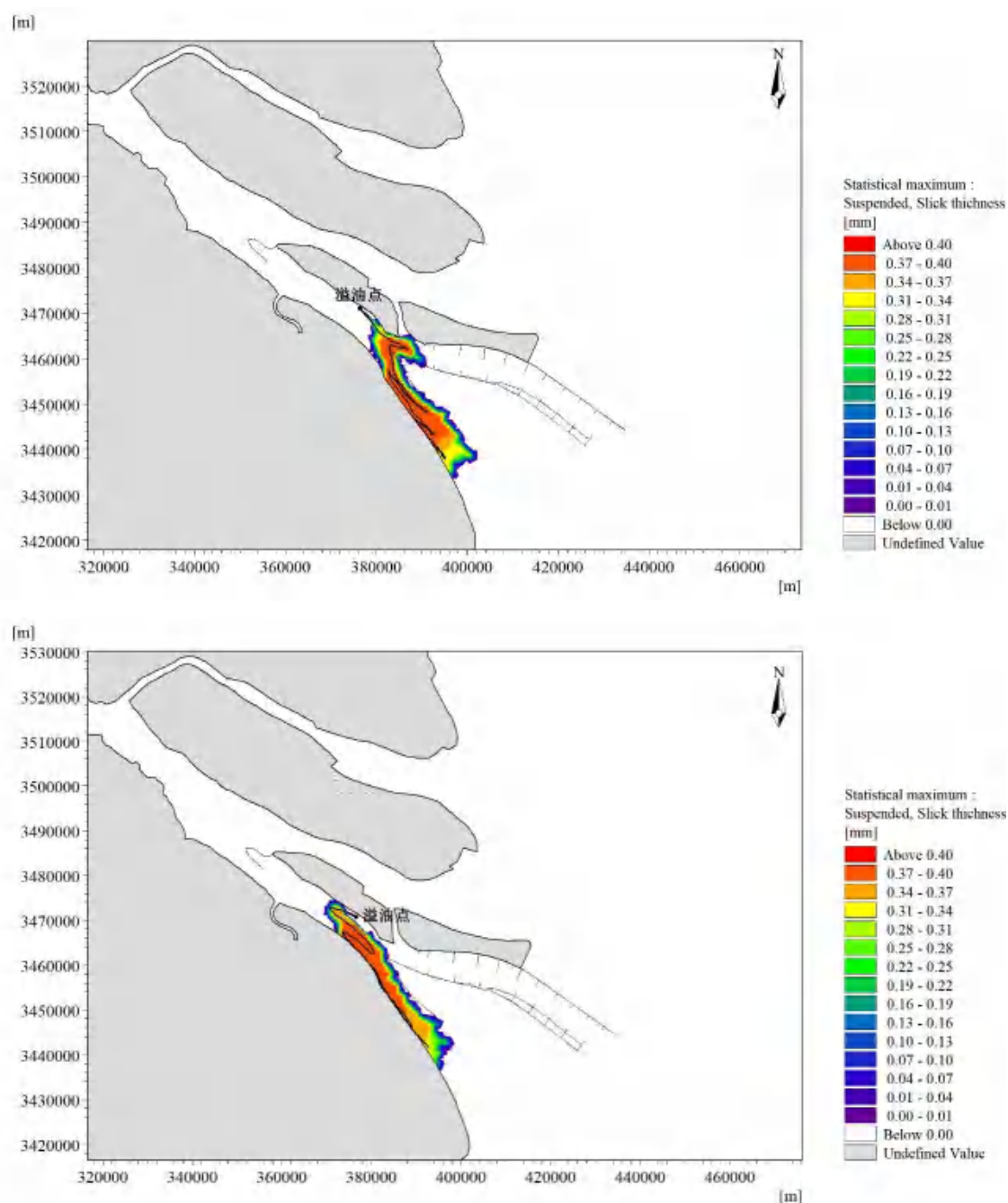
图 8.7.1-3 枯水期冬季主导风作用下油膜扫海面积和漂移轨迹图 (上为落潮时溢油, 下为涨潮时溢油, 48h)
