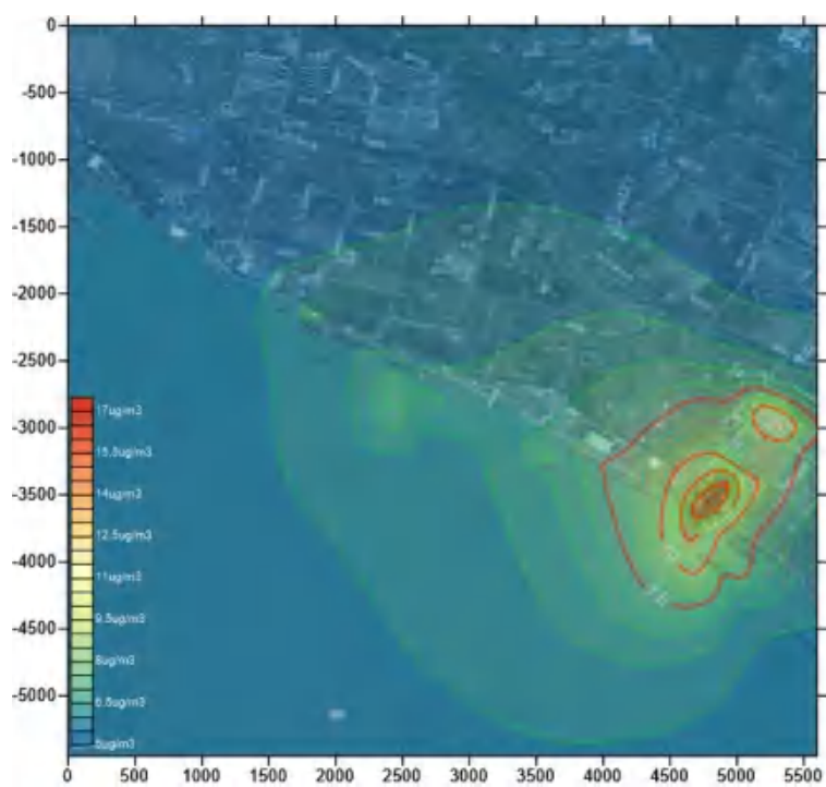
图 6.1-8 叠加现状后二甲苯小时平均浓度分布图
