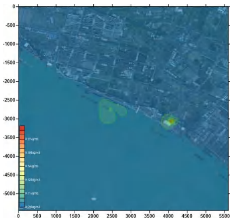
图 6.1-9 叠加现状后锰及其化合物日平均浓度分布图
