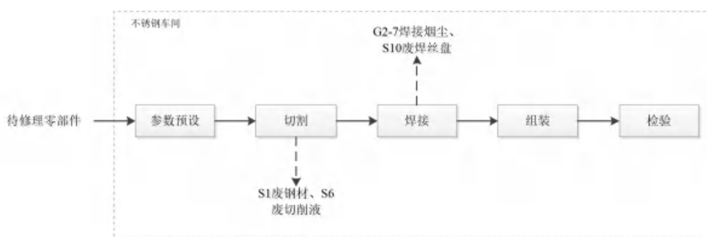
图 4.2.2-2 不锈钢件维修工艺流程及产污节点图
