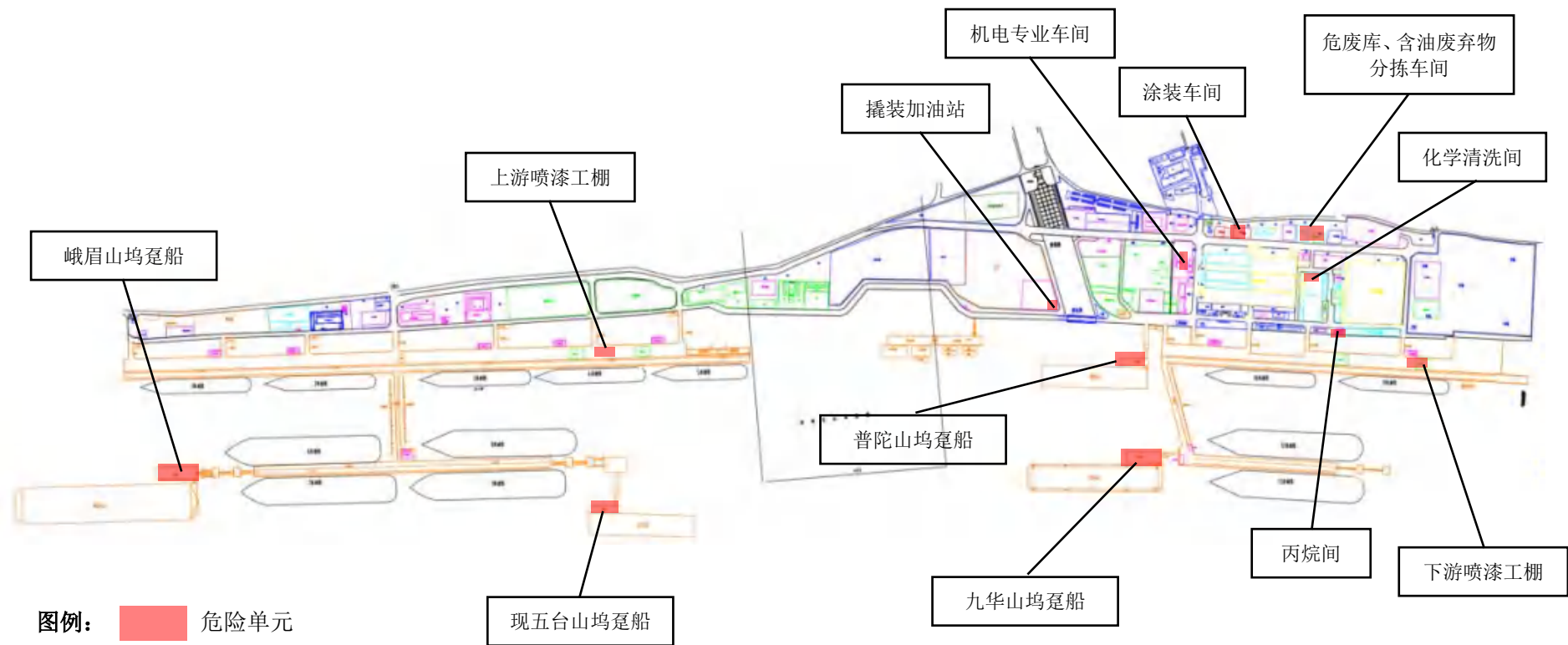
图 8.4.3-1 厂区危险单元分布图
