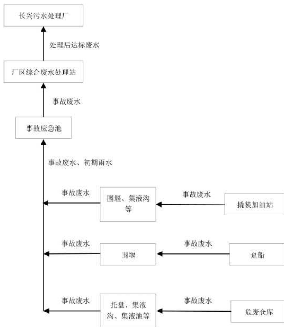
图 8.8.3-1 事故废水控制系统图
