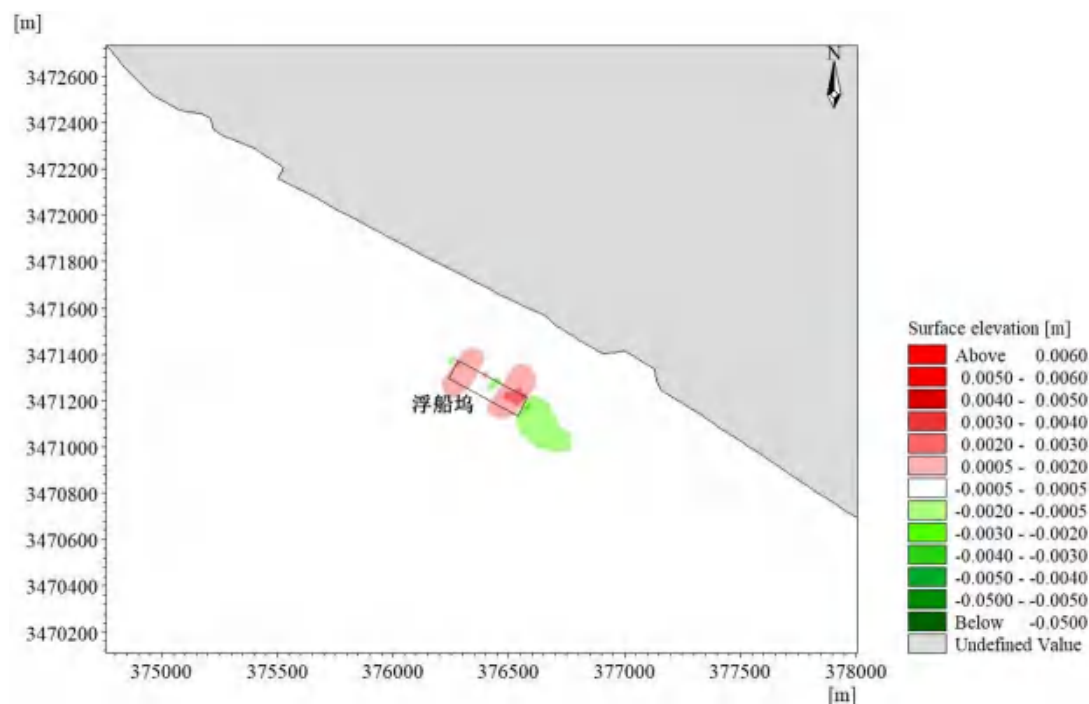
图 6.2.3-12 本工程前后涨急时刻流速大小变化图
