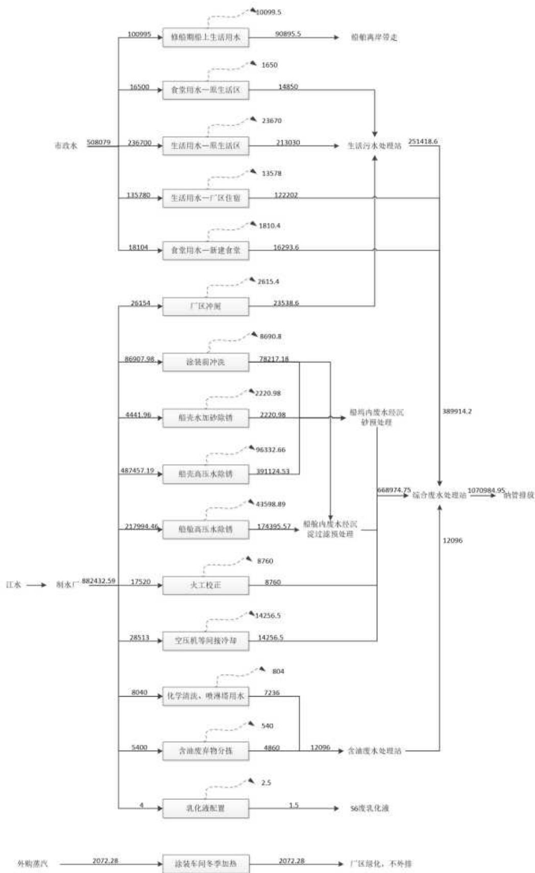
图 3.3.2-6 现有工程达纲产能水平平衡图 (单位: t/a)
