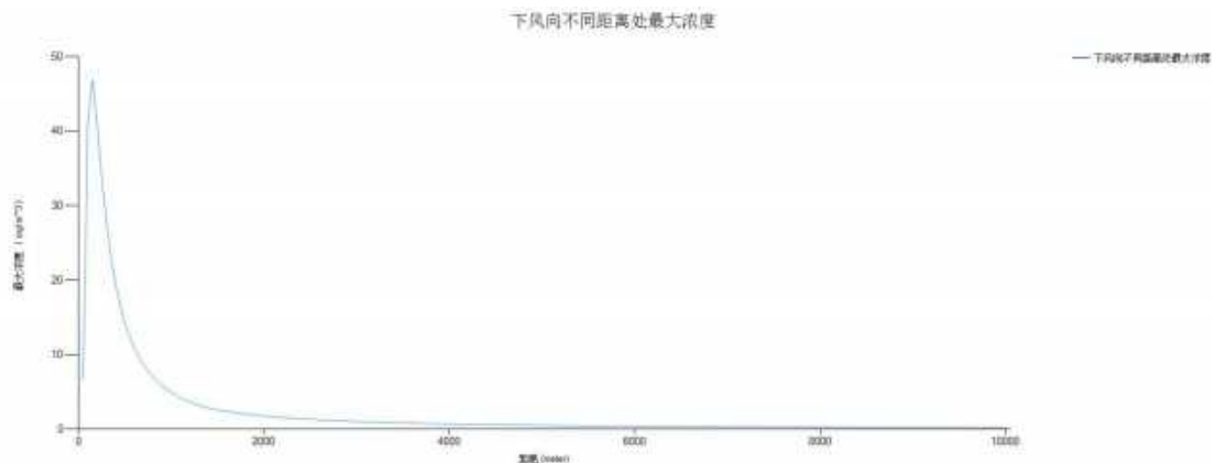
图 8.6.4-3 撬装加油站柴油火灾下风向不同距离处 CO 的最大浓度值
