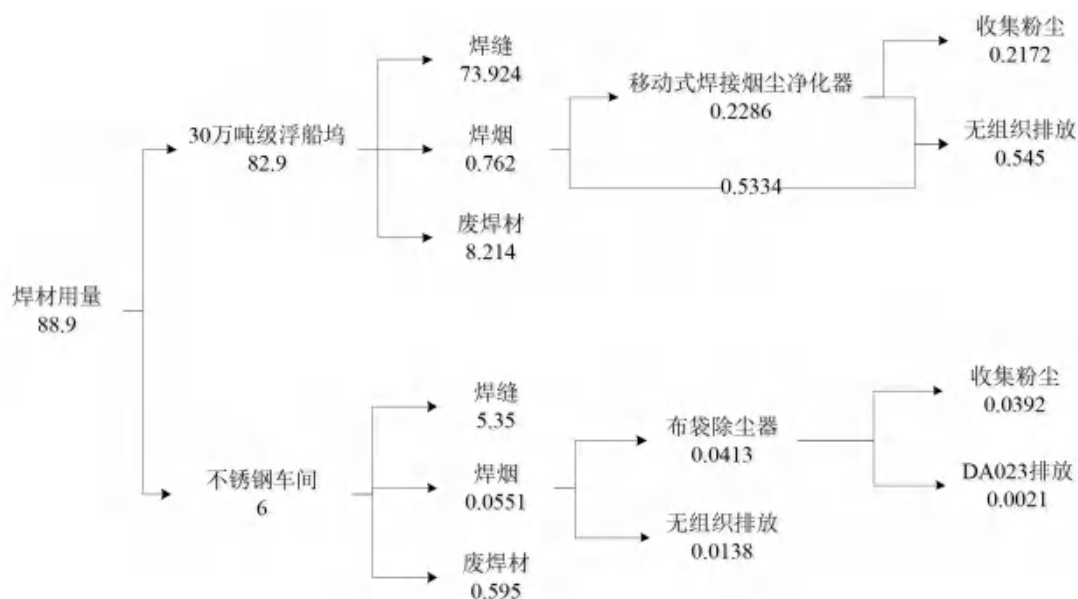
图 4.2.3-5 本工程焊材物料平衡分析图 (单位: t/a)
