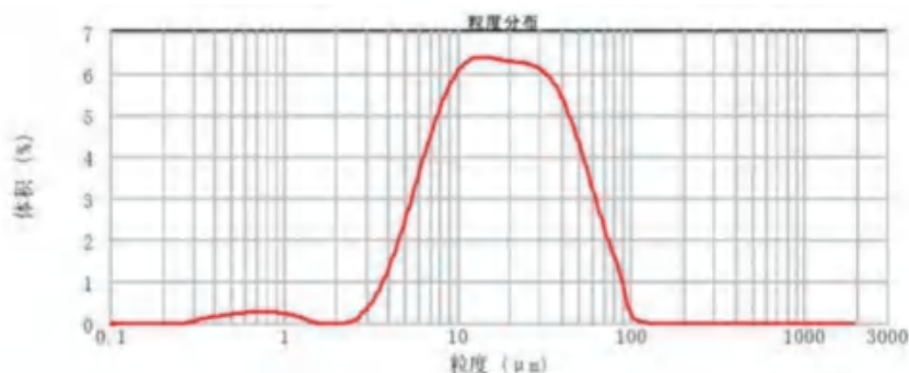
图 4.2.3-3 漆雾中不同粒径 (um) 大小油漆颗粒所占的体积百分数
