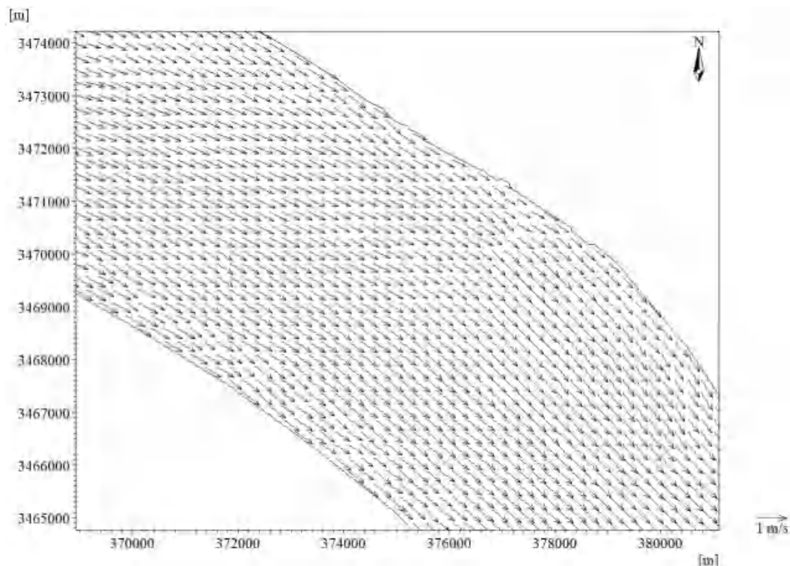
图 6.2.3-6 工程前落急流场图
