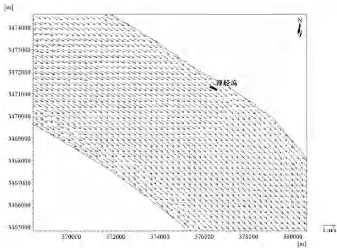
图 6.2.3-8 工程后落急流场图
