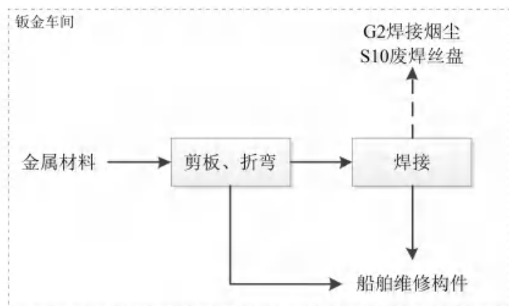
图 3.3.1-7 钣金车间生产工艺流程图
