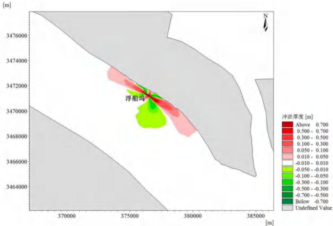
图 6.2.4-2 本工程附近冲淤平衡情况
