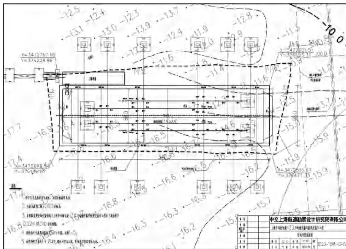
图 4.2.1-1 工程坞坑挖方范围图
