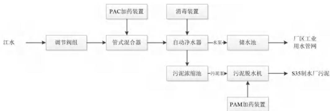
图 3.3.1-9 工业制水厂制水工艺流程图
