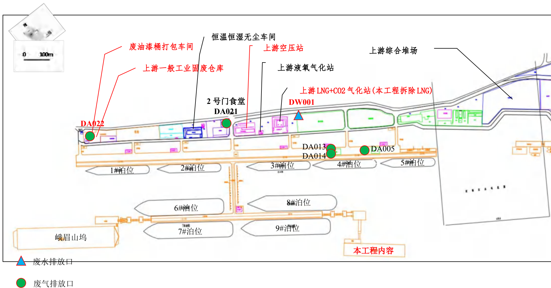
附图 11 现有工程上游厂区平面布置图
