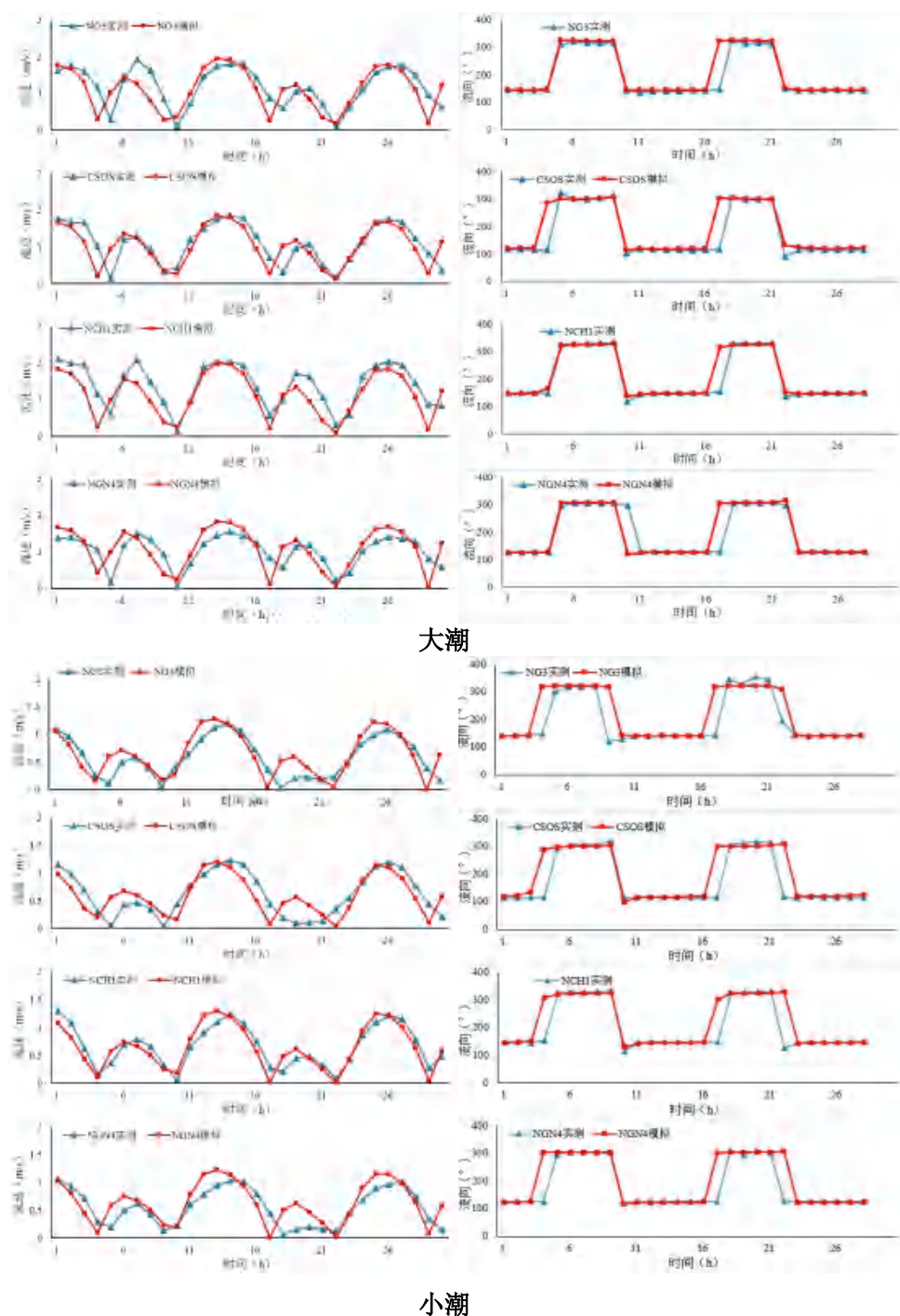
图 6.2.3-5 潮流验证图
