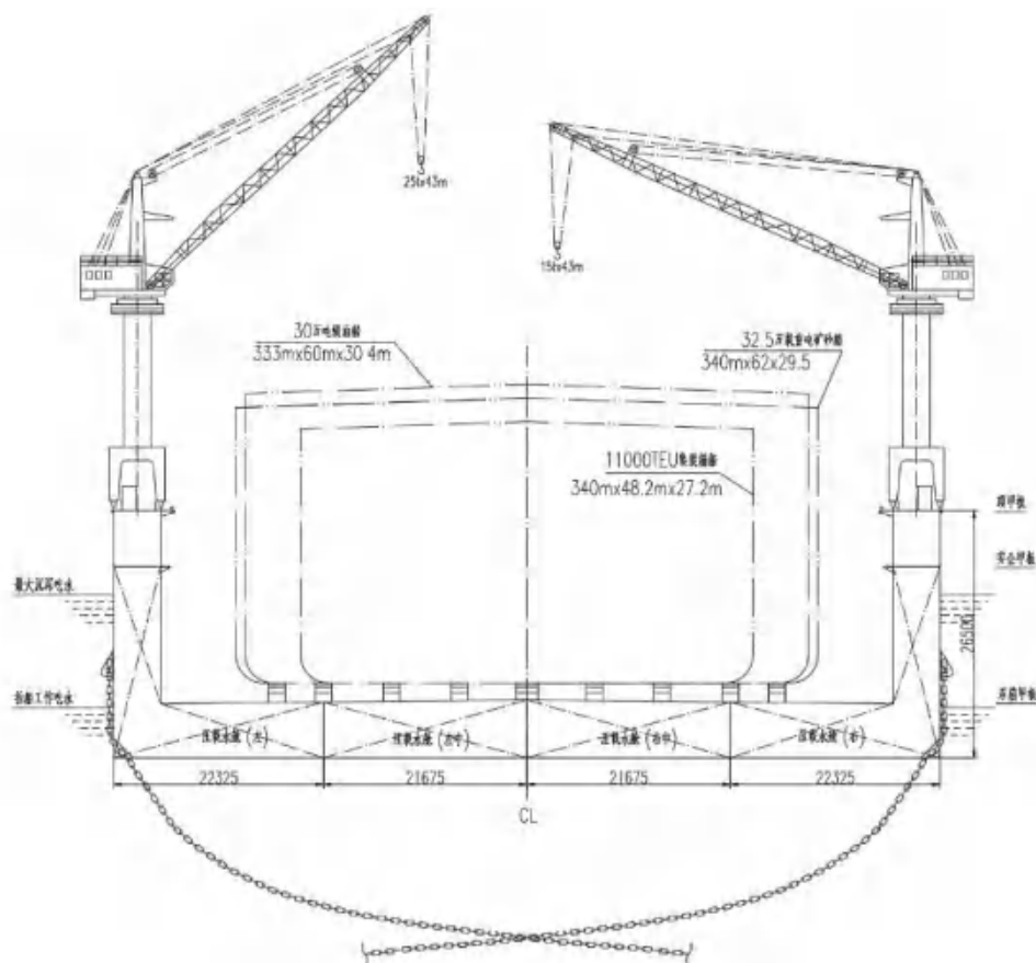
图 4.1.2-4 浮船坞断面图
