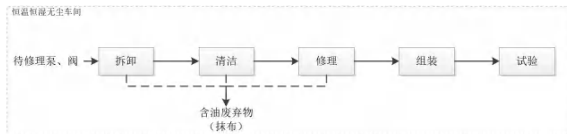
图 3.3.1-8 恒温恒湿无尘车间工艺流程图
