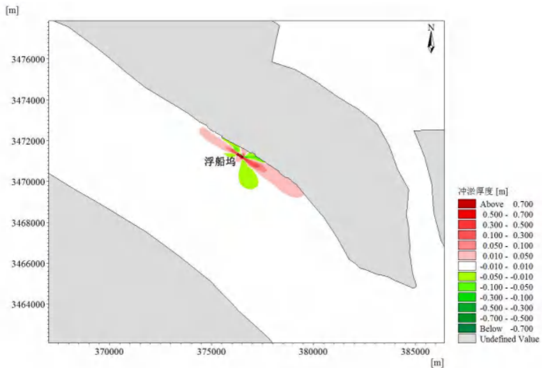
图 6.2.4-1 本工程附近冲淤情况（首年）
