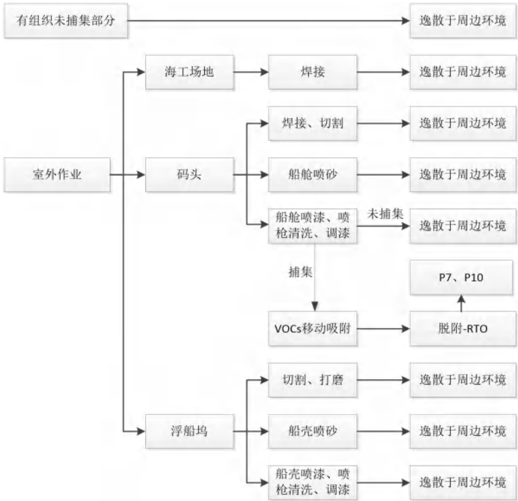
图 3.3.2-2 现有工程无组织废气处理系统图
