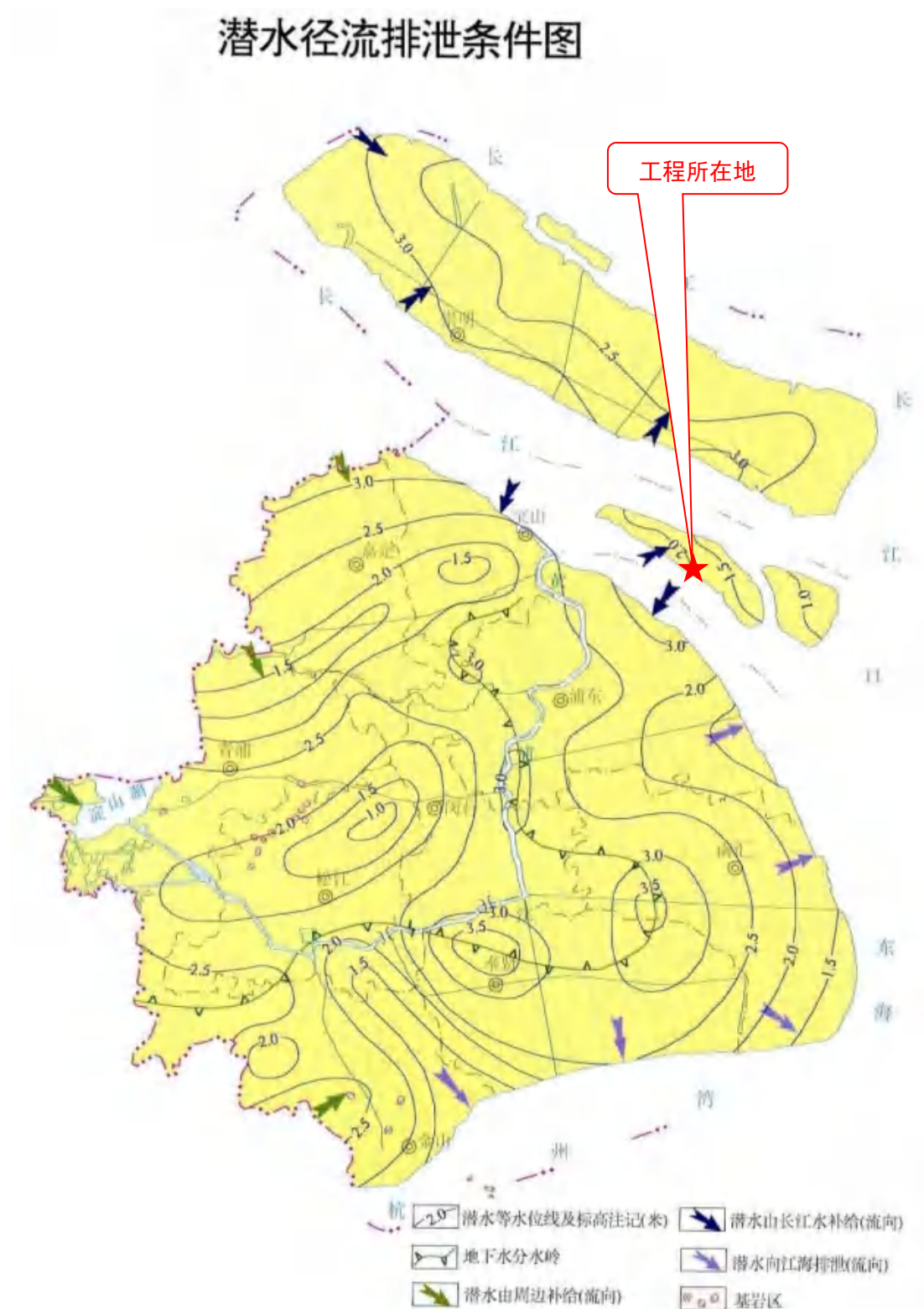
图 6.5.2-2 区域潜水径流排泄条件图
