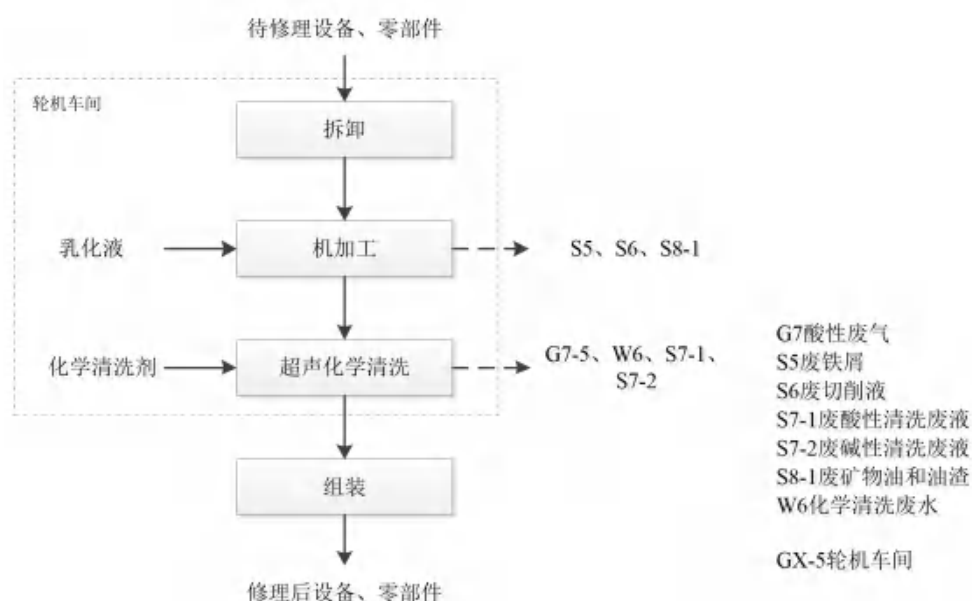
图 3.3.1-5 轮机车间生产工艺流程及产污节点图
