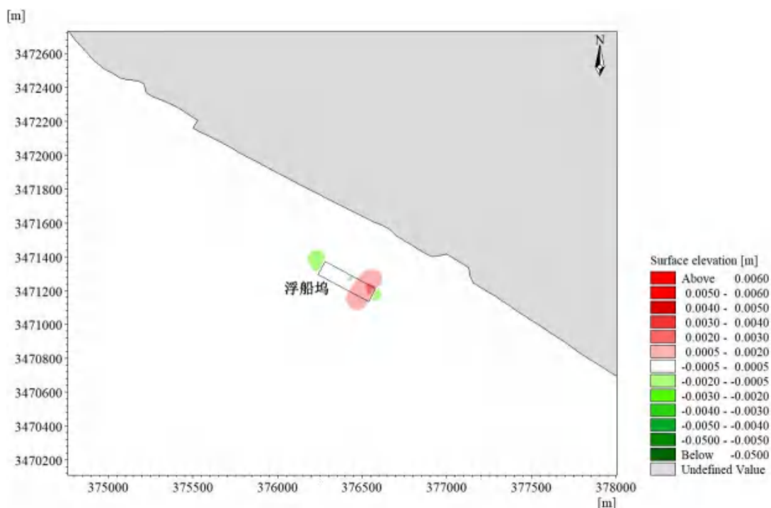
图 6.2.3-13 本工程前后涨急时刻流速大小变化图
