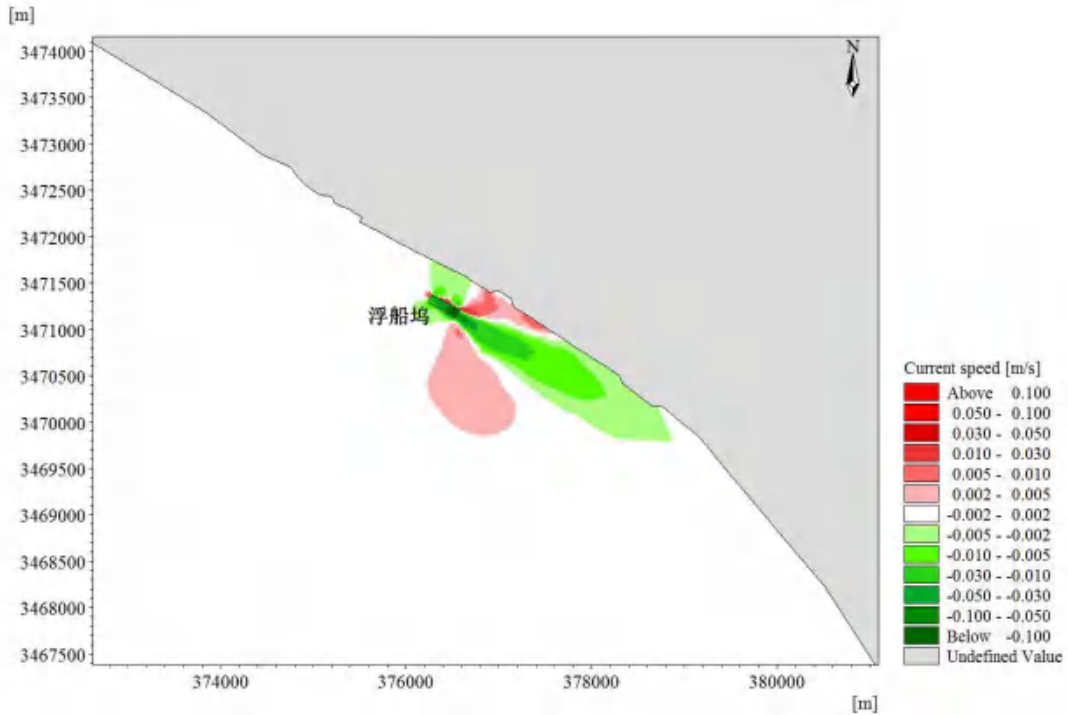
图 6.2.3-10 本工程前后落急时刻流速大小变化图
