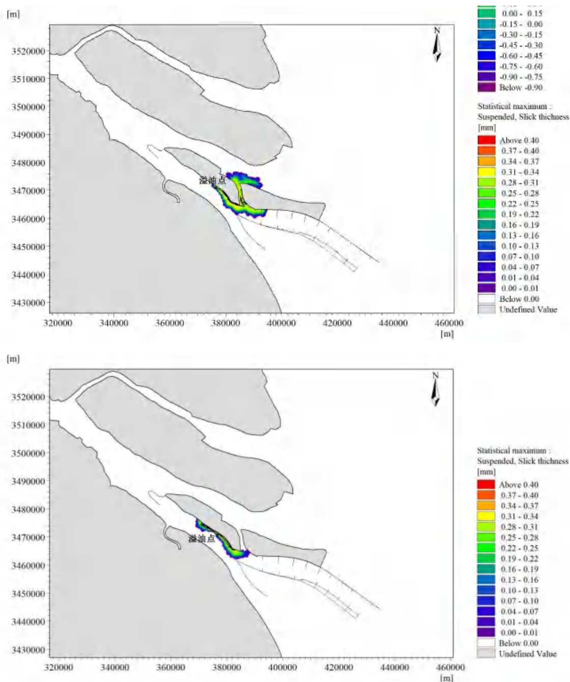
图 8.7.1-2 丰水期夏季主导风作用下油膜扫海面积和漂移轨迹图 (上为落潮时溢油, 下为涨潮时溢油, 48h)
