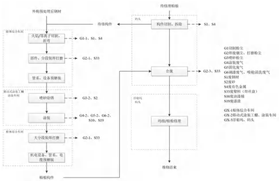
图 3.3.1-3 船舶修理流程
