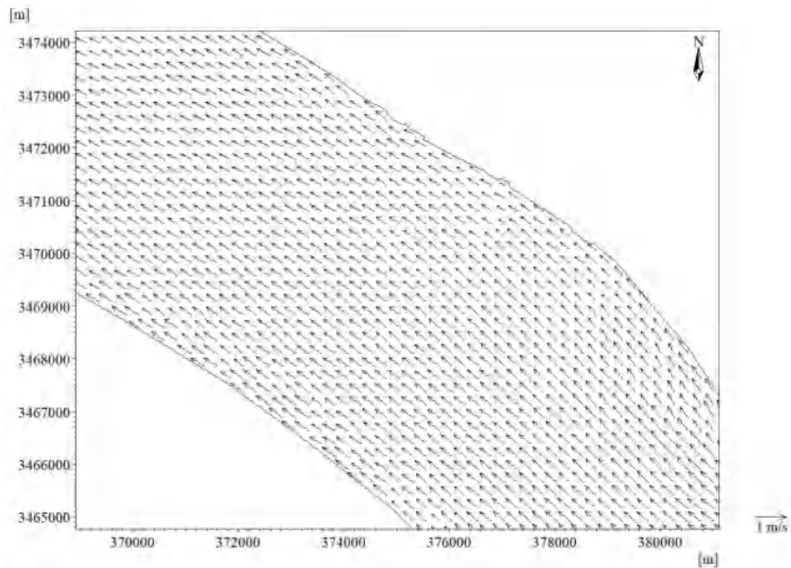
图 6.2.3-7 工程前涨急流场图
