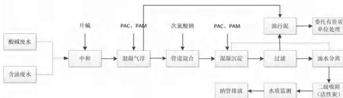
图 3.3.2-3 含油废水处理工艺流程
