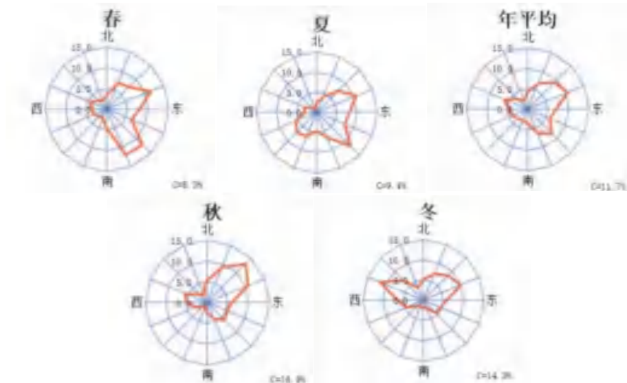
图 6.1-4 风频玫瑰图
