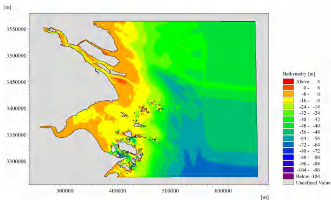
图 6.2.3-1 模拟区域地形水深示意图
