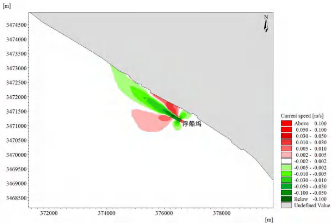
图 6.2.3-11 本工程前后涨急时刻流速大小变化图
