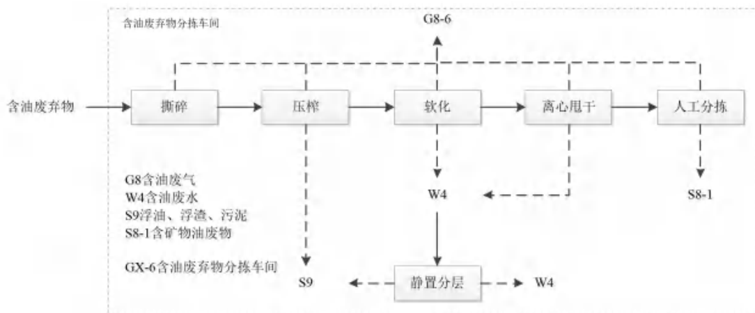
图 3.3.1-6 含油废弃物分拣工艺流程及产污节点图
