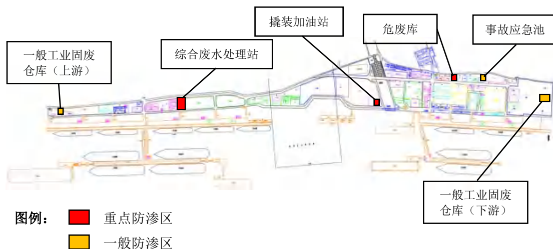
图 9.5-1 本工程防渗分区图
