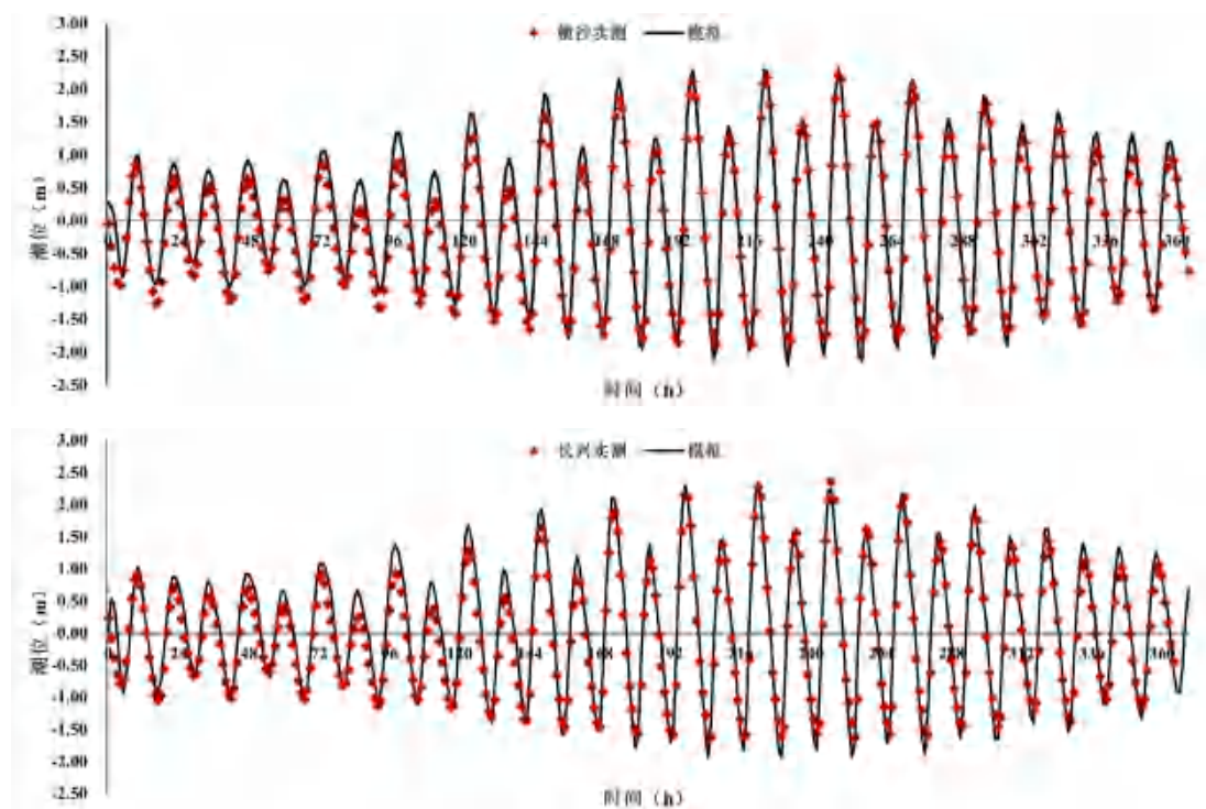
图 6.2.3-4 潮位验证图
